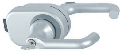
Paris vetro (chiave/nottolino) / Paris glass (key/thumbturn)
