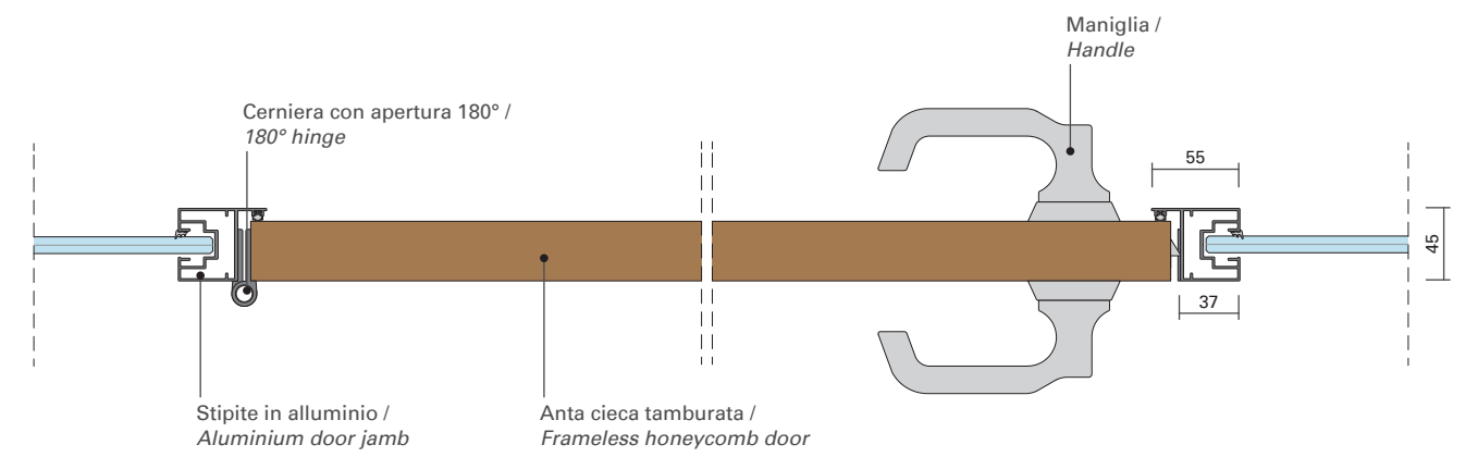
PORTA BATTENTE CIECA / FRAMELESS SWING DOOR
