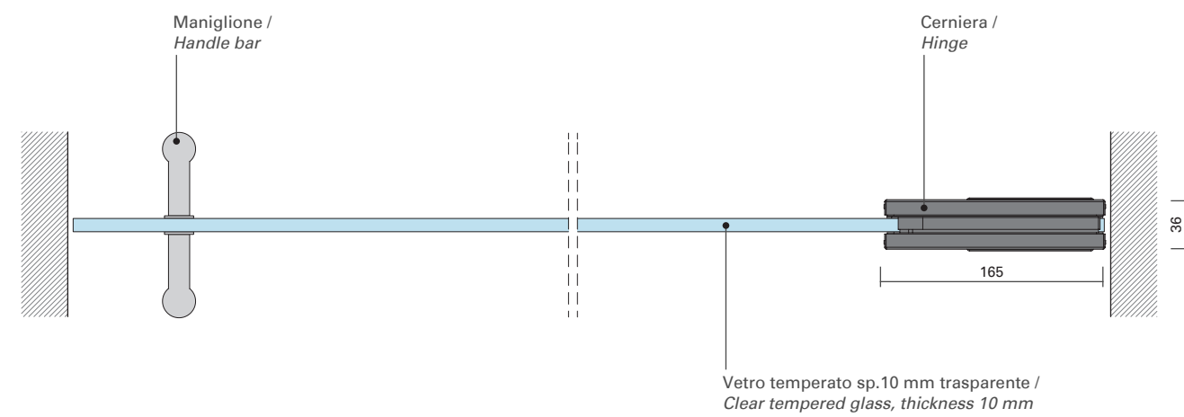
SEZIONE PORTA SINGOLA VA VIENI SU MURATURA / DOUBLE-ACTING DOOR SECTION ON MASONRY WALL
