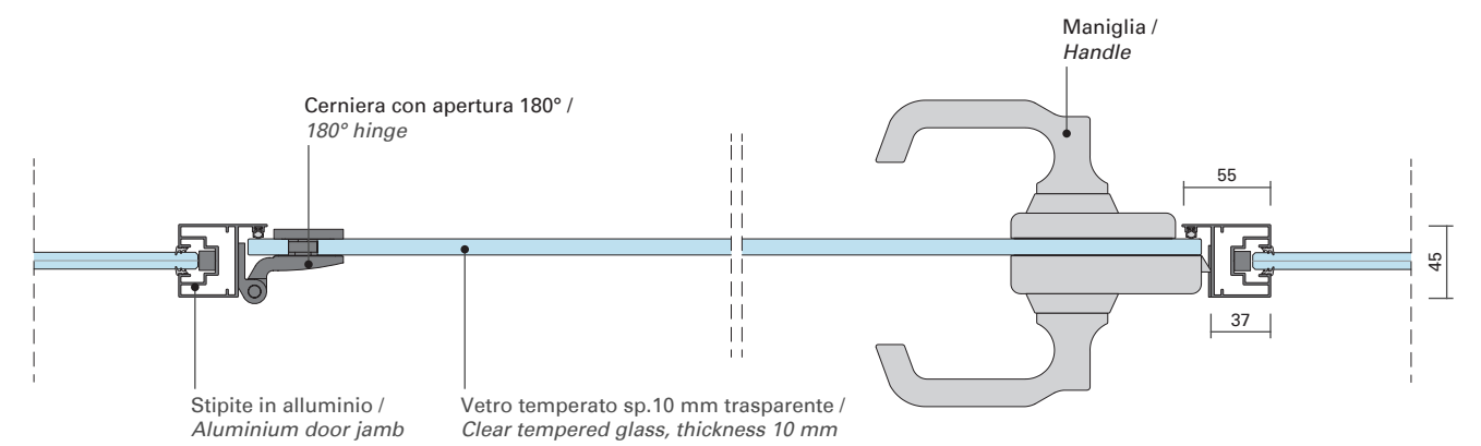
PORTA BATTENTE VETRATA FILO LUCIDO / SWING GLASS DOOR WITH POLISHED EDGE
