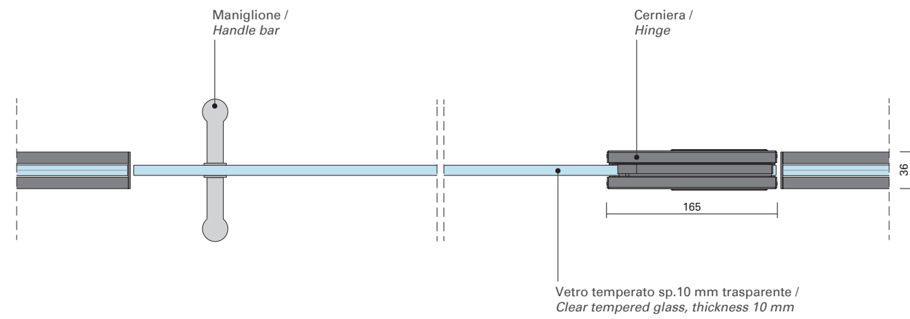
SEZIONE PORTA SINGOLA VA VIENI SU PARETE VETRATA / DOUBLE-ACTING DOOR SECTION ON GLAZED PARTITION
